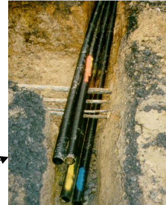
MSH Außenansicht und Schutzrohrbündel im gemeinsamen Rohrgraben
