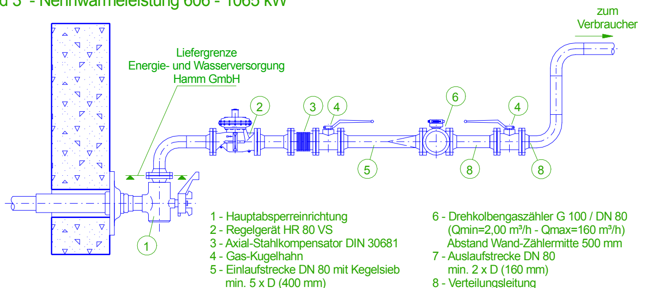
Bild 3 - Nennwärmeleistung 606 - 1065 kW
