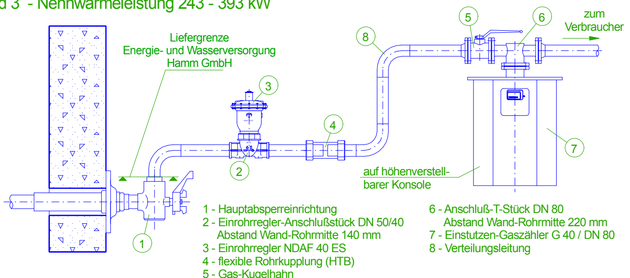
Bild 3 - Nennwärmeleistung 243 - 393 kW
