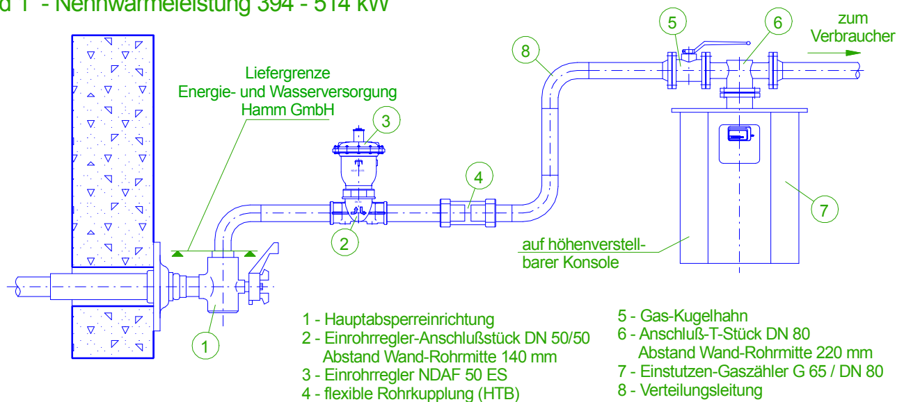
Bild 2 - Nennwärmeleistung 515 - 605 kW
