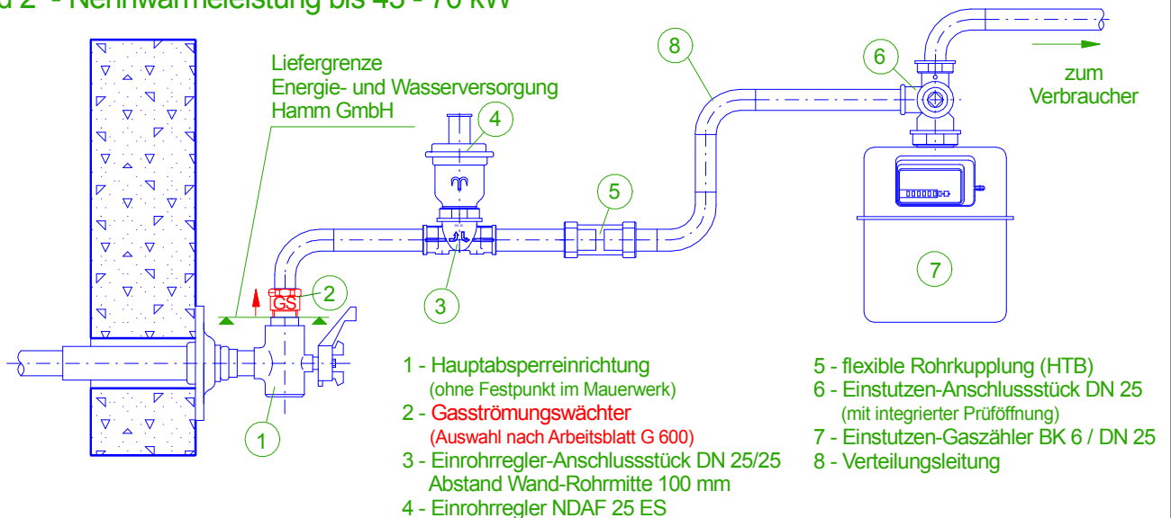
Bild 3 - Nennwärmeleistung 71 - 97 kW
