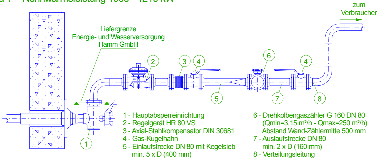
Bild 1 - Nennwärmeleistung 1066 - 1210 kW
