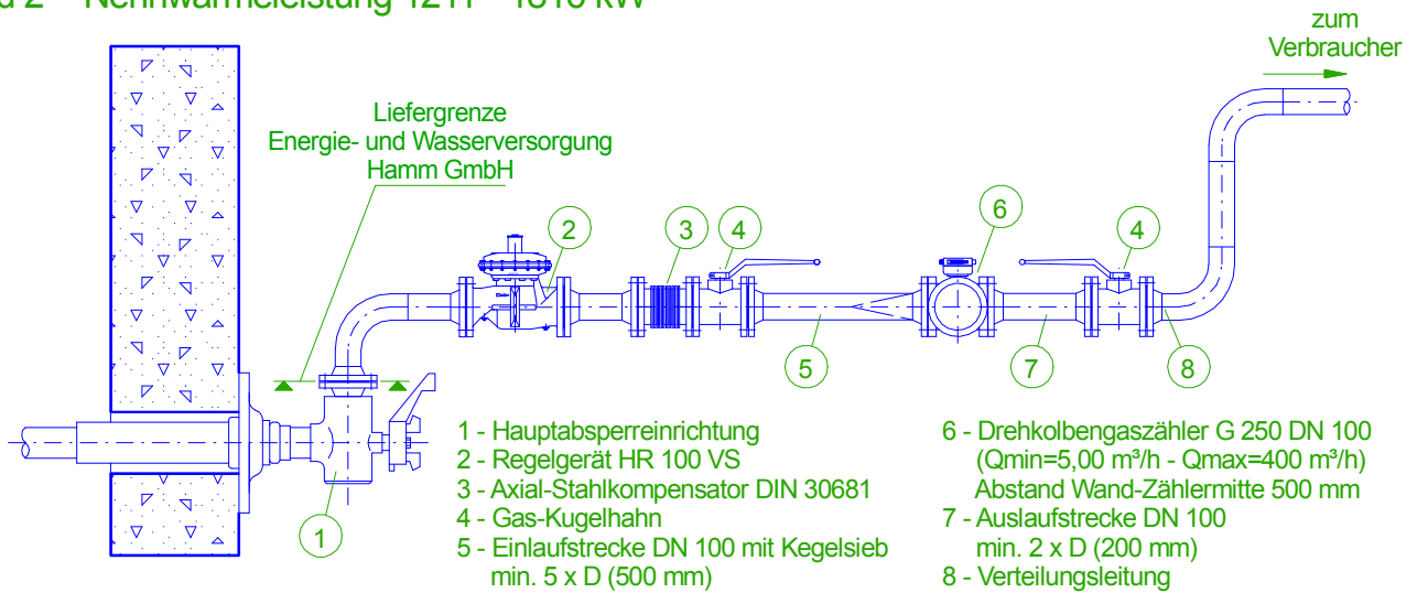
Bild 2 - Nennwärmeleistung 1211 - 1816 kW
