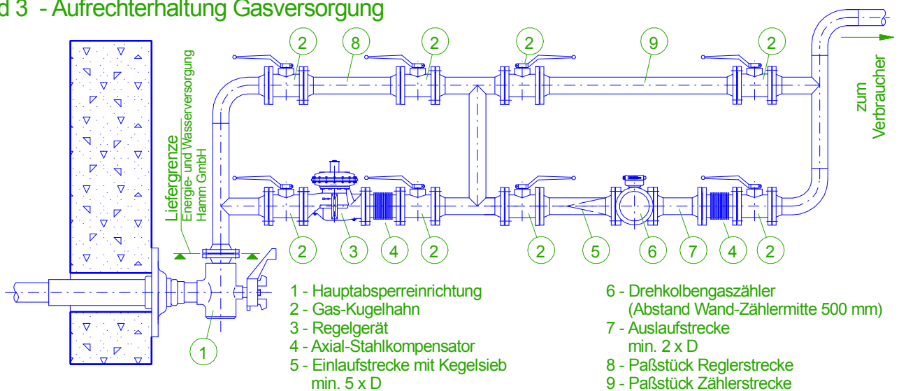
Bild 3 - Aufrechterhaltung Gasversorgung
