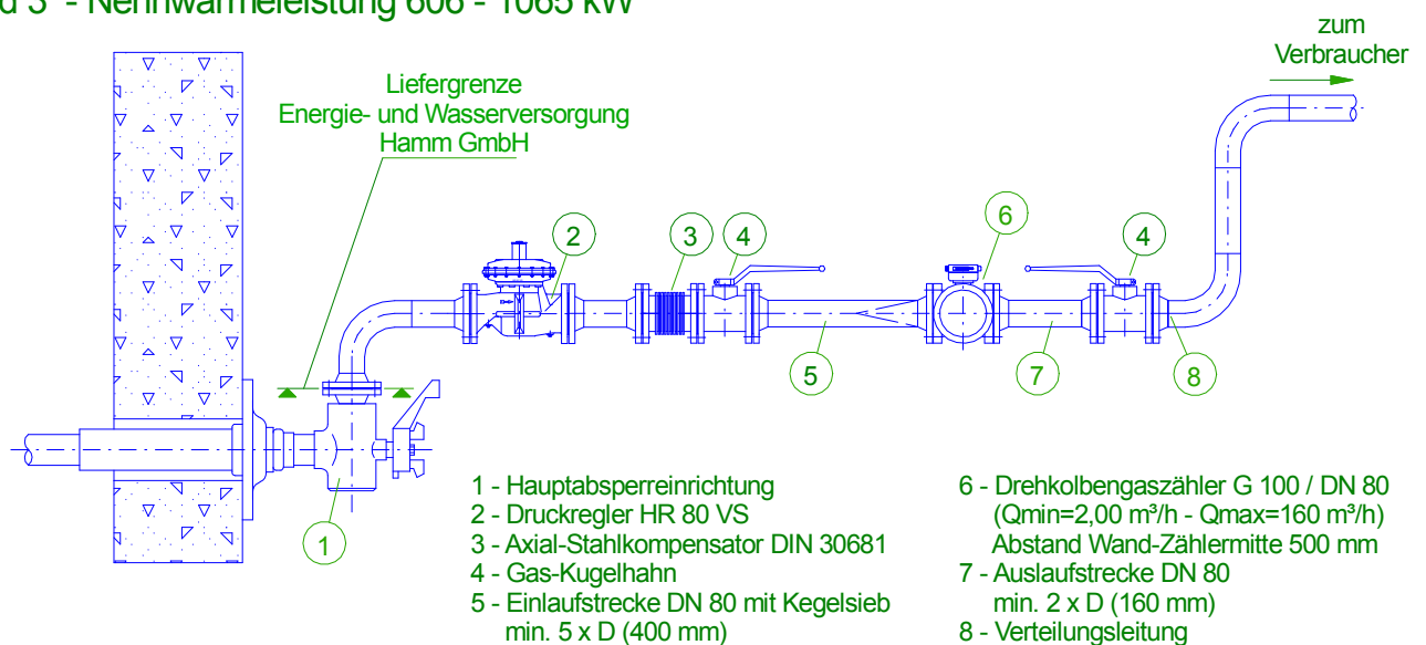
Bild 3 - Nennwärmeleistung 606 - 1065 kW
