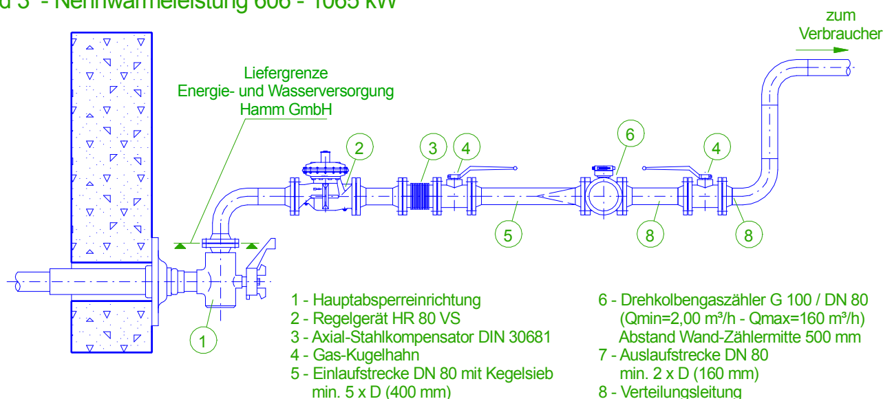
Bild 3 - Nennwärmeleistung 606 - 1065 kW
